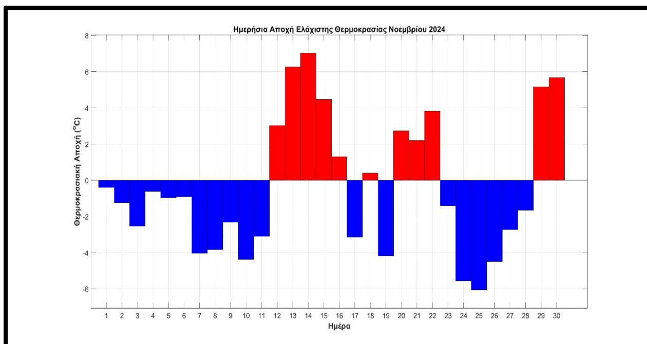
Σχήμα 4. Αποχές (με κόκκινο χρώμα οι θετικές και με μπλε οι αρνητικές) των φετινών από τις μέσες κλιματικές τιμές της ελάχιστης ημερήσιας θερμοκρασίας στα Ιωάννινα για το μήνα Νοέμβριο του 2024.
