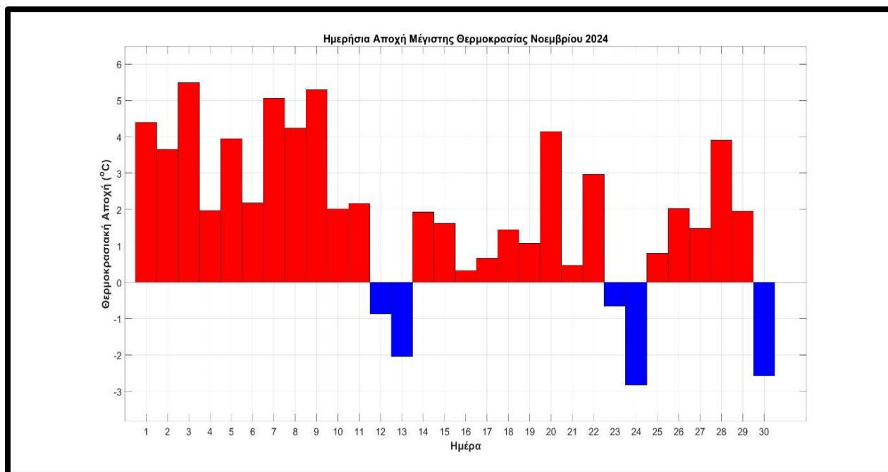
Σχήμα 2. Αποχές (με κόκκινο χρώμα οι θετικές και με μπλε οι αρνητικές) των φετινών από τις μέσες κλιματικές τιμές της μέγιστης ημερήσιας θερμοκρασίας στα Ιωάννινα για το μήνα Νοέμβριο του 2024.
