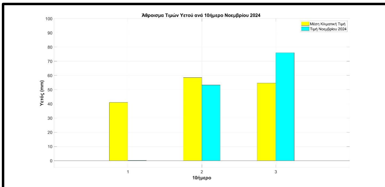
Σχήμα 10. Διακύμανση των αθροιστικών τιμών υετού ανά δεκαήμερο στα Ιωάννινα για το μήνα Νοέμβριο κατά το έτος 2024. Οι κίτρινες στήλες δείχνουν τις μέσες κλιματικές τιμές, ενώ οι γαλάζιες στήλες τις φετινές τιμές.
