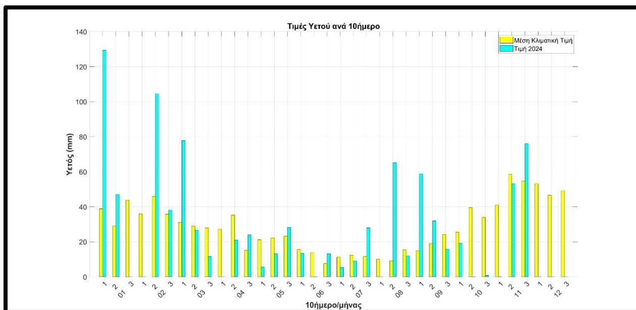
Σχήμα 13. Διακύμανση των αθροιστικών τιμών υετού ανά δεκαήμερο στα Ιωάννινα (έως και το μήνα Νοέμβριο) κατά το έτος 2024. Οι κίτρινες στήλες δείχνουν τις μέσες κλιματικές τιμές, ενώ οι γαλάζιες στήλες τις φετινές τιμές.
