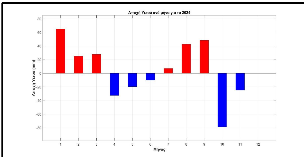
Σχήμα 16. Διακύμανση των αποχών ανά μήνα (με κόκκινο χρώμα οι θετικές και με μπλε οι αρνητικές) του υετού στα Ιωάννινα (έως και το μήνα Νοέμβριο) κατά το έτος 2024.
