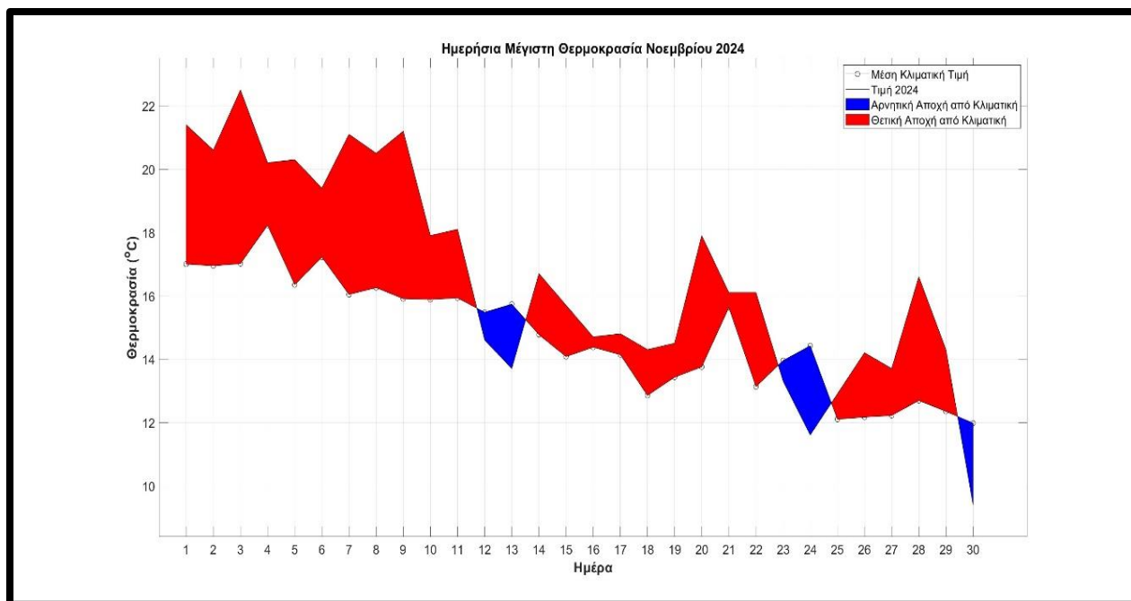
Σχήμα 1. Τιμές μέγιστης ημερήσιας θερμοκρασίας στα Ιωάννινα για τον Νοέμβριο του 2024 και αντίστοιχες μέσες κλιματικές τιμές για τον ίδιο μήνα. Με κόκκινο χρώμα φαίνονται οι θετικές αποχές (διαφορές) των φετινών τιμών από τις κλιματικές, ενώ με μπλε χρώμα οι αρνητικές αποχές.
