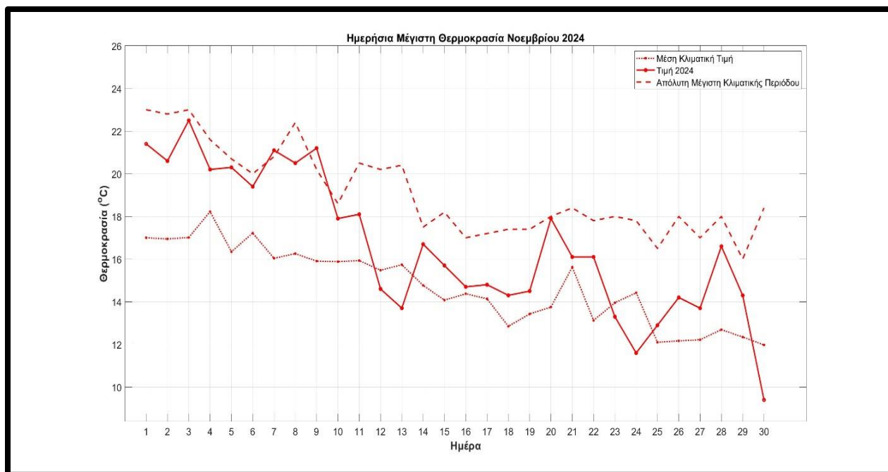
Σχήμα 5. Διακύμανση της μέγιστης ημερήσιας θερμοκρασίας στα Ιωάννινα κατά το μήνα Νοέμβριο του 2024. Η διάστικτη καμπύλη δείχνει τις μέσες κλιματικές τιμές, η διακεκομμένη καμπύλη δείχνει τις απόλυτες μέγιστες τιμές και η συνεχής καμπύλη με τα σημεία δείχνει τις φετινές τιμές.
