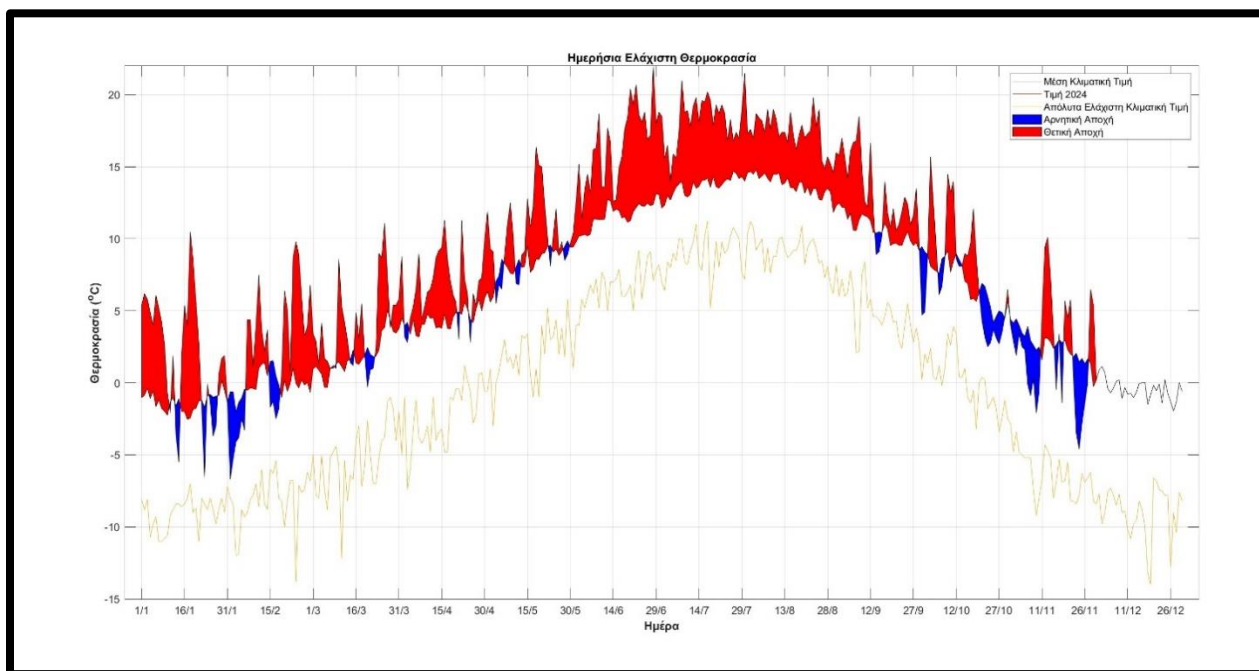
Σχήμα 8. Διακύμανση της ελάχιστης ημερήσιας θερμοκρασίας στα Ιωάννινα (έως και το μήνα Νοέμβριο) κατά το έτος 2024. Η μπλε/μαύρη καμπύλη δείχνει τις μέσες κλιματικές τιμές, η πορτοκαλί καμπύλη δείχνει τις απόλυτες ελάχιστες.
