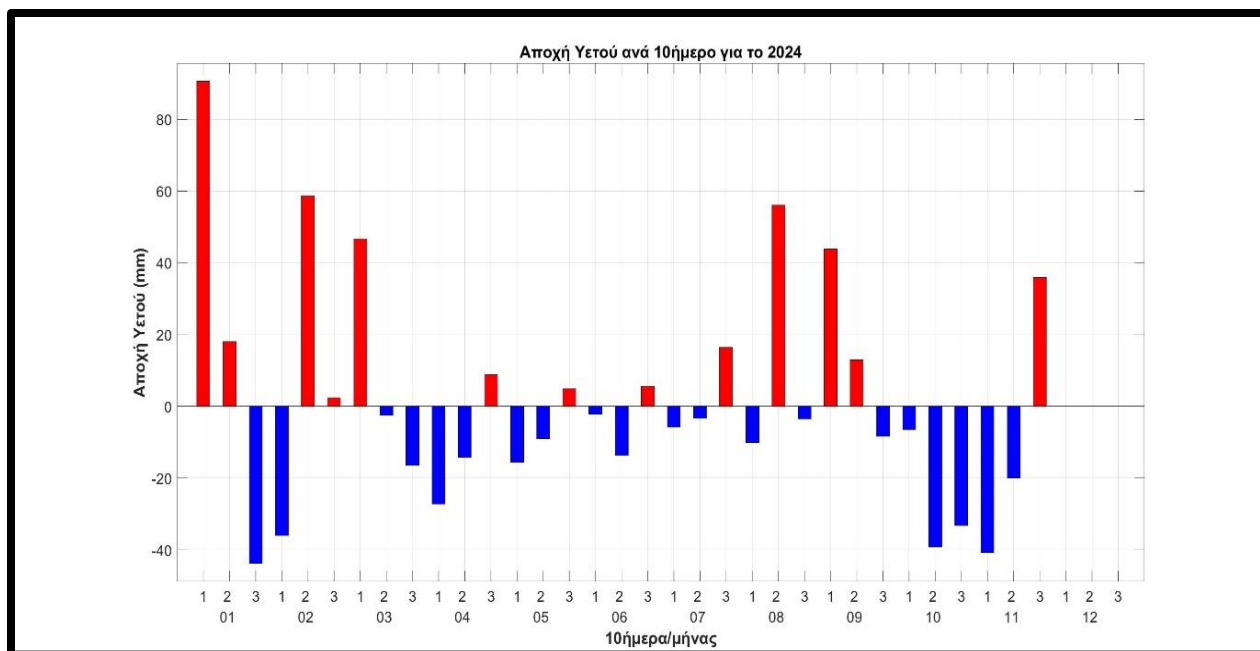
Σχήμα 14. Διακύμανση των αποχών ανά δεκαήμερο (με κόκκινο χρώμα οι θετικές και με μπλε οι αρνητικές) του υετού στα Ιωάννινα (έως και το μήνα Νοέμβριο) κατά το έτος 2024.
