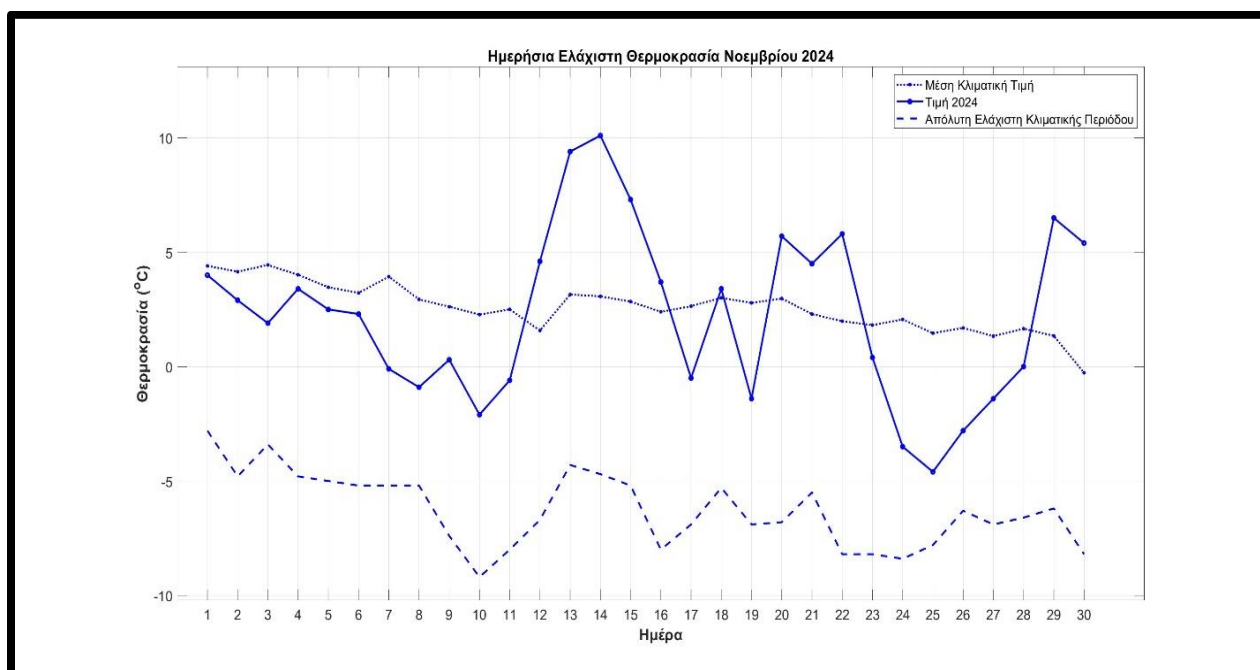
Σχήμα 6. Διακύμανση της ελάχιστης ημερήσιας θερμοκρασίας στα Ιωάννινα κατά το μήνα Νοέμβριο του 2024. Η διάστικτη καμπύλη δείχνει τις μέσες κλιματικές τιμές, η διακεκομμένη καμπύλη δείχνει τις απόλυτες ελάχιστες τιμές και η συνεχής καμπύλη με τα σημεία δείχνει τις φετινές τιμές.
