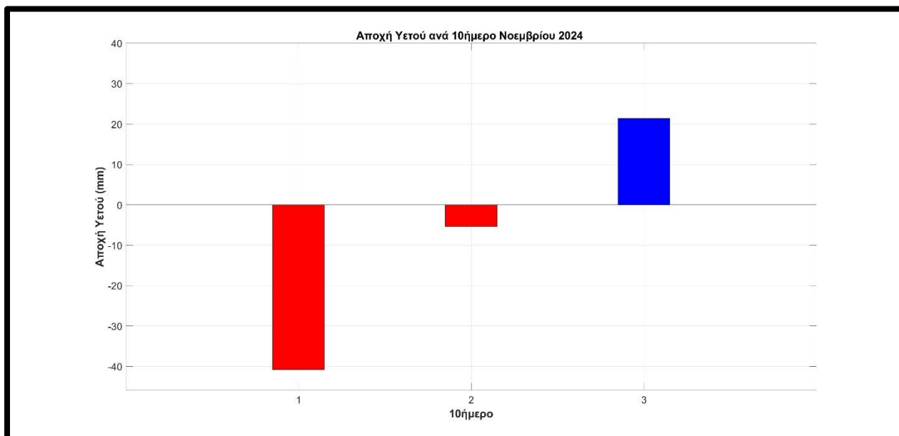
Σχήμα 11. Αποχές (με κόκκινο χρώμα οι θετικές και με μπλε οι αρνητικές) των φετινών από τις μέσες κλιματικές τιμές των τιμών υετού στα Ιωάννινα για το μήνα Νοέμβριο, 2024.
