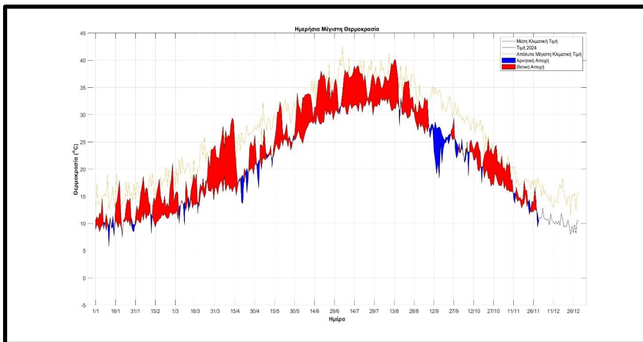
Σχήμα 7. Διακύμανση της μέγιστης ημερήσιας θερμοκρασίας στα Ιωάννινα (έως και το μήνα Νοέμβριο) κατά το έτος 2024. Η μπλε/μαύρη καμπύλη δείχνει τις μέσες κλιματικές τιμές, η πορτοκαλί καμπύλη δείχνει τις απόλυτες μέγιστες τιμές.
