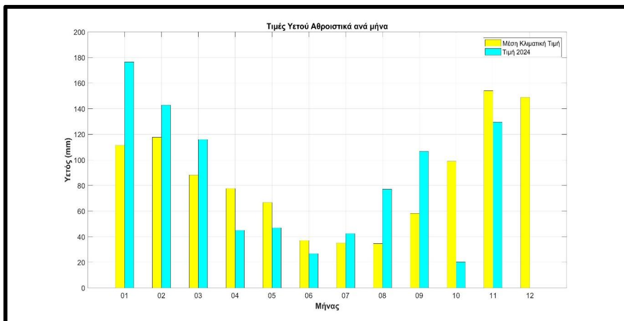
Σχήμα 15. Διακύμανση των τιμών υετού αθροιστικά ανά μήνα στα Ιωάννινα (έως και το μήνα Νοέμβριο) κατά το έτος 2024. Η κίτρινη μπάρα δείχνει τις μέσες κλιματικές τιμές, ενώ η γαλάζια μπάρα δείχνει τις φετινές τιμές.
