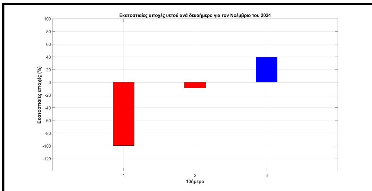
Σχήμα 12. Εκατοστιαίες απόλυτες αποχές (με κόκκινο χρώμα οι θετικές και με μπλε οι αρνητικές) ανά δεκαήμερο για τον μήνα Νοέμβριο, 2024.
