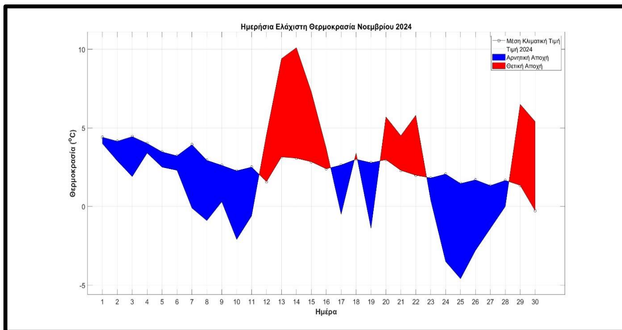
Σχήμα 3. Τιμές ελάχιστης ημερήσιας θερμοκρασίας στα Ιωάννινα για τον Νοέμβριο του 2024 και αντίστοιχες μέσες κλιματικές τιμές για τον ίδιο μήνα. Με κόκκινο χρώμα φαίνονται οι θετικές αποχές (διαφορές) των φετινών τιμών από τις κλιματικές, ενώ με μπλε χρώμα οι αρνητικές αποχές.
