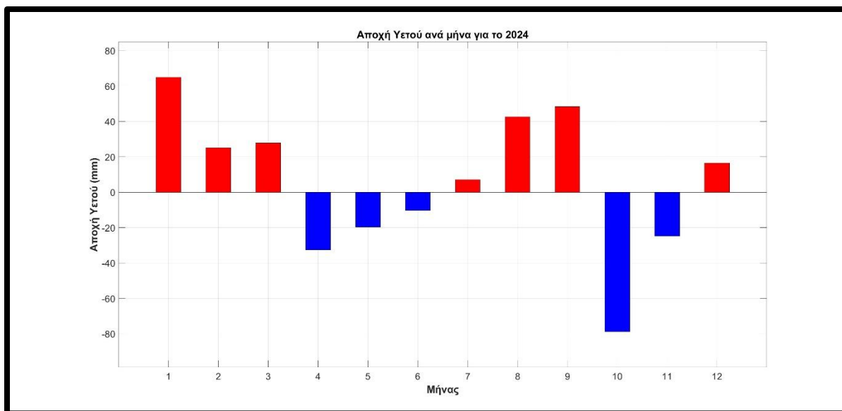
Σχήμα 16. Διακύμανση των αποχών ανά μήνα (με κόκκινο χρώμα οι θετικές και με μπλε οι αρνητικές) του υετού στα Ιωάννινα (έως και το μήνα Δεκέμβριο) κατά το έτος 2024.
