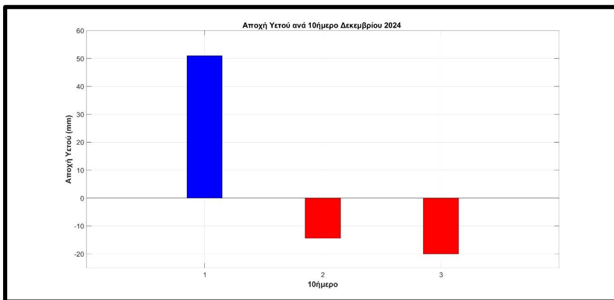
Σχήμα 11. Αποχές (με κόκκινο χρώμα οι θετικές και με μπλε οι αρνητικές) των φετινών από τις μέσες κλιματικές τιμές των τιμών υετού στα Ιωάννινα για το μήνα Δεκέμβριο, 2024.
