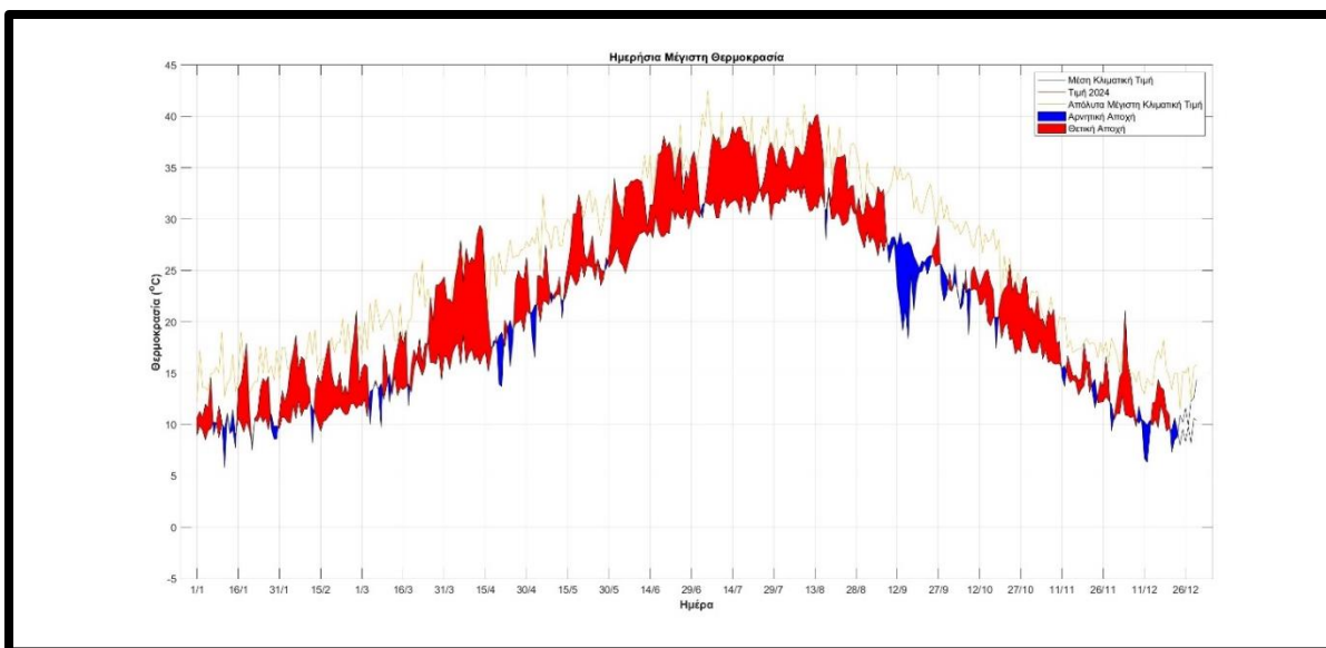
Σχήμα 7. Διακύμανση της μέγιστης ημερήσιας θερμοκρασίας στα Ιωάννινα (έως και το μήνα Δεκέμβριο) κατά το έτος 2024. Η μπλε/μαύρη καμπύλη δείχνει τις μέσες κλιματικές τιμές, η πορτοκαλί καμπύλη δείχνει τις απόλυτες μέγιστες τιμές.
