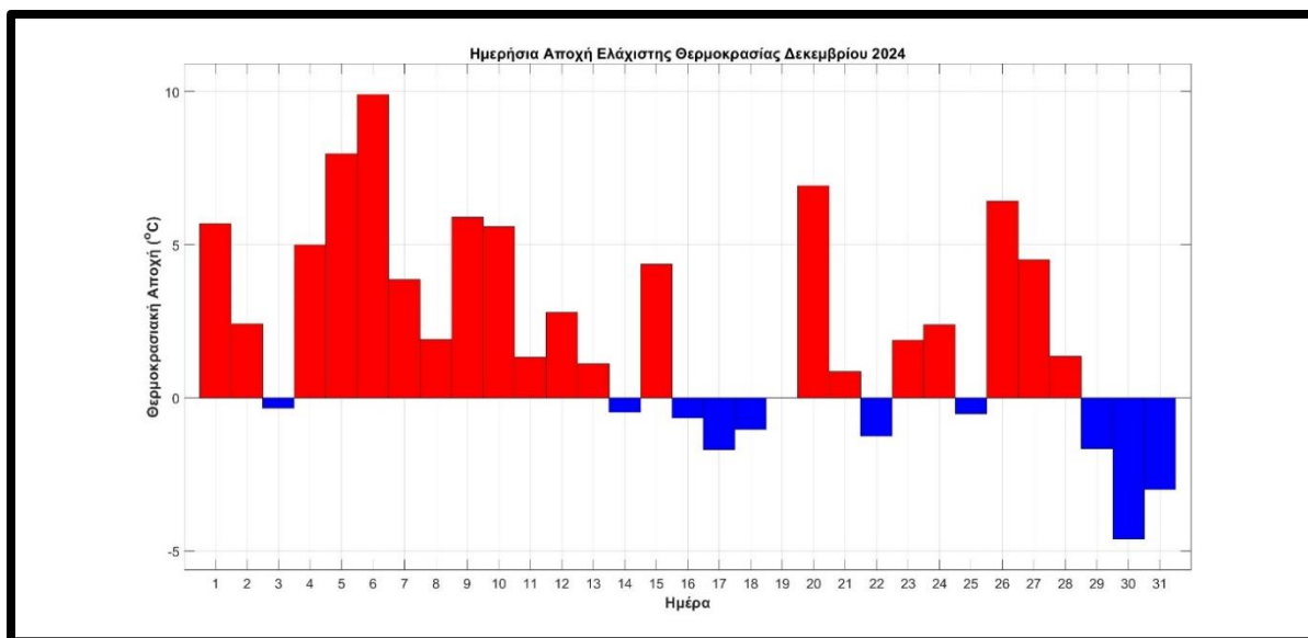
Σχήμα 4. Αποχές (με κόκκινο χρώμα οι θετικές και με μπλε οι αρνητικές) των φετινών από τις μέσες κλιματικές τιμές της ελάχιστης ημερήσιας θερμοκρασίας στα Ιωάννινα για το μήνα Δεκέμβριο του 2024.
