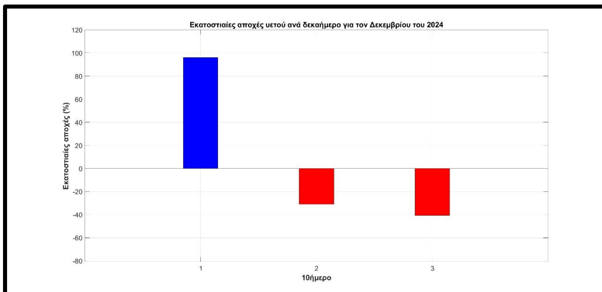
Σχήμα 12. Εκατοστιαίες απόλυτες αποχές (με κόκκινο χρώμα οι θετικές και με μπλε οι αρνητικές) ανά δεκαήμερο για τον μήνα Δεκέμβριο, 2024.
