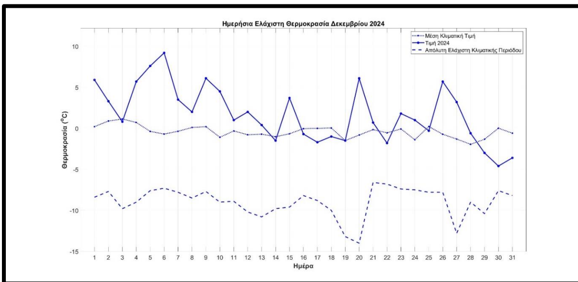
Σχήμα 6. Διακύμανση της ελάχιστης ημερήσιας θερμοκρασίας στα Ιωάννινα κατά το μήνα Δεκέμβριο του 2024. Η διάστικτη καμπύλη δείχνει τις μέσες κλιματικές τιμές, η διακεκομμένη καμπύλη δείχνει τις απόλυτες ελάχιστες τιμές και η συνεχής καμπύλη με τα σημεία δείχνει τις φετινές τιμές.
