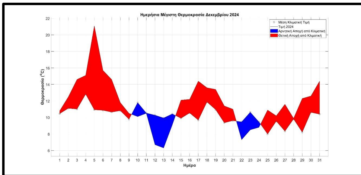
Σχήμα 1. Τιμές μέγιστης ημερήσιας θερμοκρασίας στα Ιωάννινα για τον Δεκέμβριο του 2024 και αντίστοιχες μέσες κλιματικές τιμές για τον ίδιο μήνα. Με κόκκινο χρώμα φαίνονται οι θετικές αποχές (διαφορές) των φετινών τιμών από τις κλιματικές, ενώ με μπλε χρώμα οι αρνητικές αποχές.
