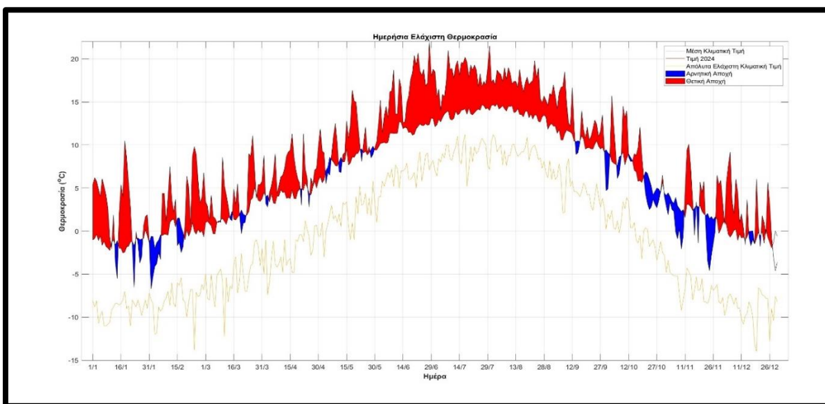
Σχήμα 8. Διακύμανση της ελάχιστης ημερήσιας θερμοκρασίας στα Ιωάννινα (έως και το μήνα Δεκέμβριο) κατά το έτος 2024. Η μπλε/μαύρη καμπύλη δείχνει τις μέσες κλιματικές τιμές, η πορτοκαλί καμπύλη δείχνει τις απόλυτες ελάχιστες τιμές.
