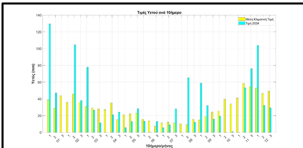
Σχήμα 13. Διακύμανση των αθροιστικών τιμών υετού ανά δεκαήμερο στα Ιωάννινα (έως και το μήνα Δεκέμβριο) κατά το έτος 2024. Οι κίτρινες στήλες δείχνουν τις μέσες κλιματικές τιμές, ενώ οι γαλάζιες στήλες τις φετινές τιμές.
