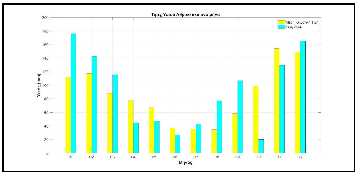
Σχήμα 15. Διακύμανση των τιμών υετού αθροιστικά ανά μήνα στα Ιωάννινα (έως και το μήνα Δεκέμβριο) κατά το έτος 2024. Η κίτρινη μπάρα δείχνει τις μέσες κλιματικές τιμές, ενώ η γαλάζια μπάρα δείχνει τις φετινές τιμές.
