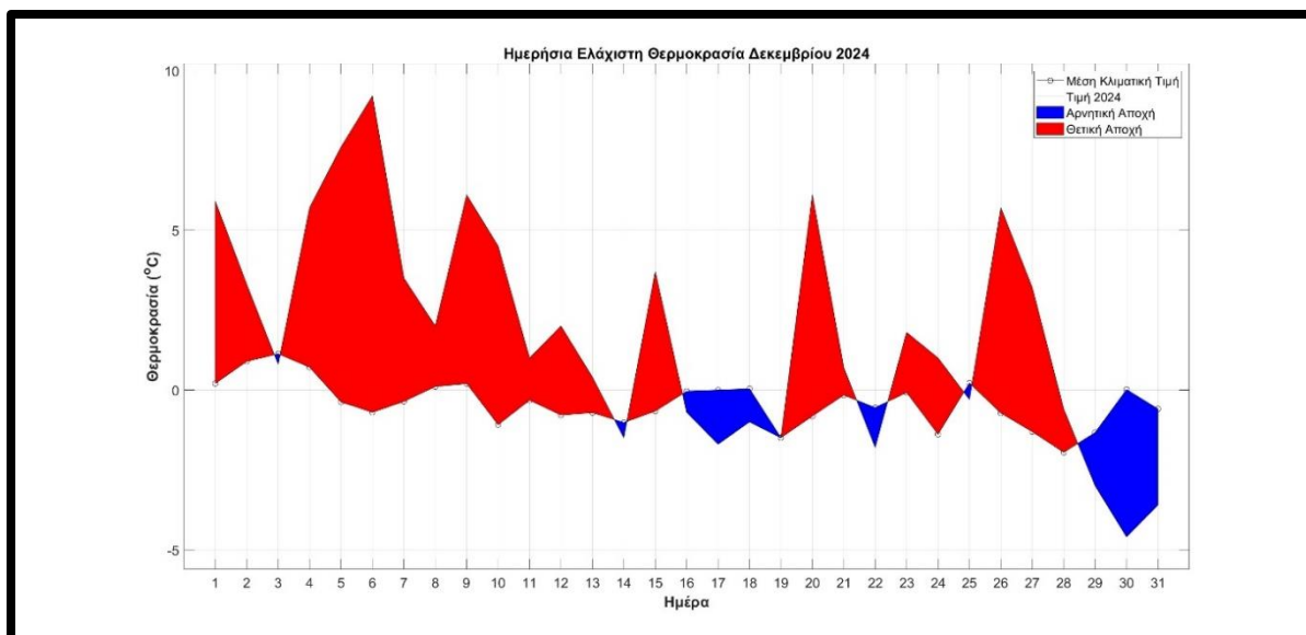
Σχήμα 3. Τιμές ελάχιστης ημερήσιας θερμοκρασίας στα Ιωάννινα για τον Δεκέμβριο του 2024 και αντίστοιχες μέσες κλιματικές τιμές για τον ίδιο μήνα. Με κόκκινο χρώμα φαίνονται οι θετικές αποχές (διαφορές) των φετινών τιμών από τις κλιματικές, ενώ με μπλε χρώμα οι αρνητικές αποχές.
