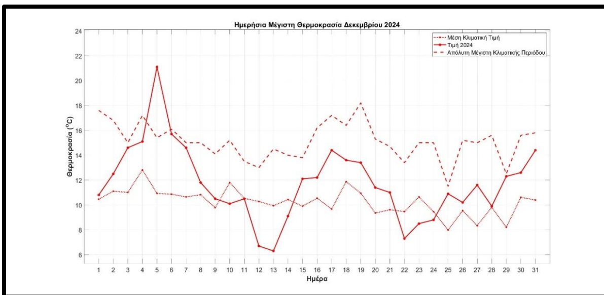
Σχήμα 5. Διακύμανση της μέγιστης ημερήσιας θερμοκρασίας στα Ιωάννινα κατά το μήνα Δεκέμβριο του 2024. Η διάστικτη καμπύλη δείχνει τις μέσες κλιματικές τιμές, η διακεκομμένη καμπύλη δείχνει τις απόλυτες μέγιστες τιμές και η συνεχής καμπύλη με τα σημεία δείχνει τις φετινές τιμές.
