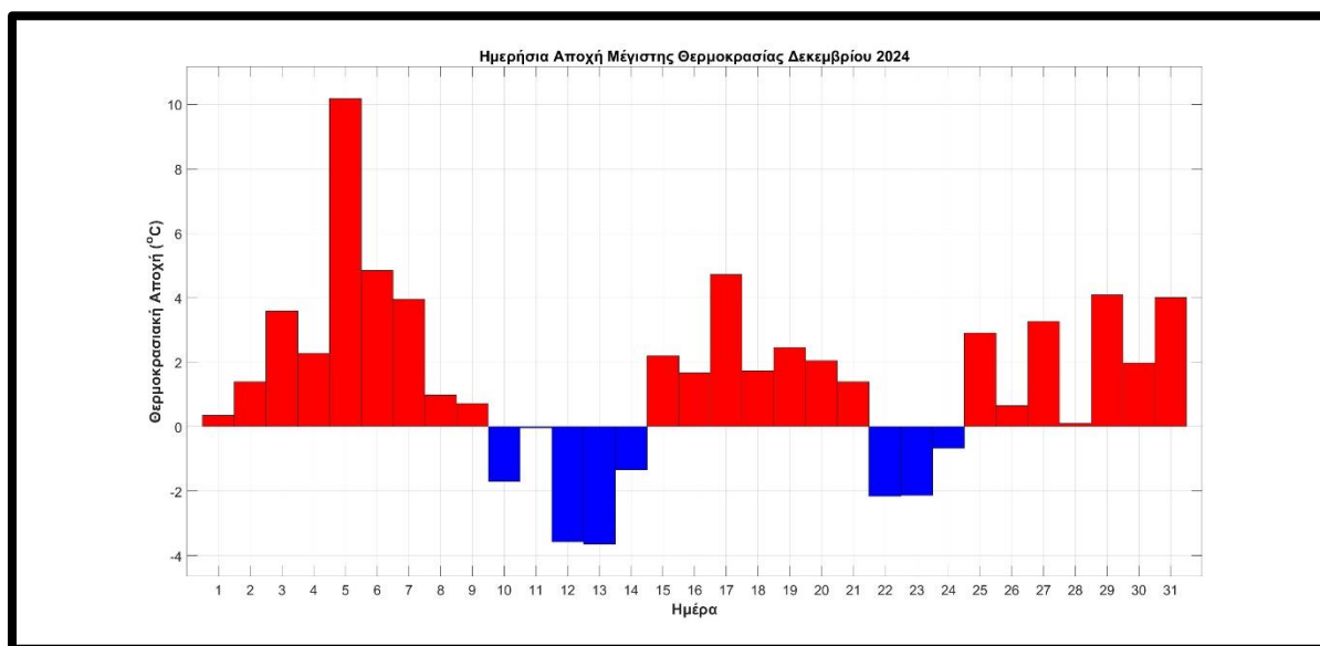
Σχήμα 2. Αποχές (με κόκκινο χρώμα οι θετικές και με μπλε οι αρνητικές) των φετινών από τις μέσες κλιματικές τιμές της μέγιστης ημερήσιας θερμοκρασίας στα Ιωάννινα για το μήνα Δεκέμβριο του 2024.
