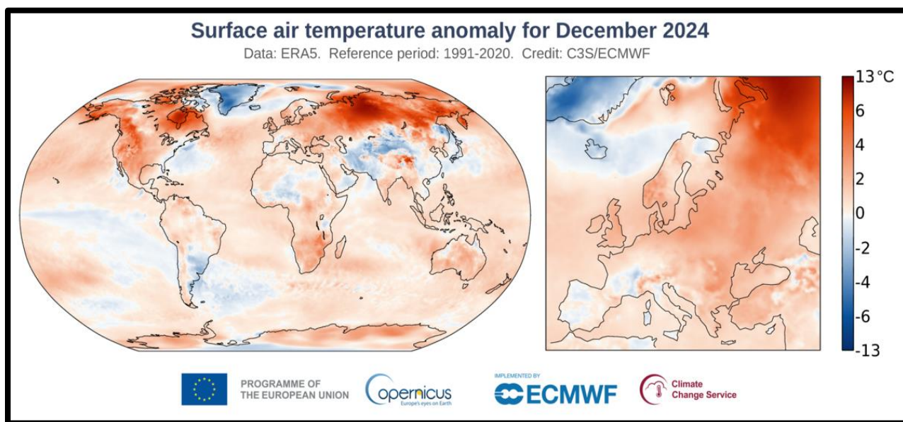
Σχήμα 9. Ανωμαλία (αποχή) της επιφανειακής θερμοκρασίας για τη Γη (αριστερά) και την Ευρώπη (δεξιά) κατά τον Δεκέμβριο του 2024 (Πηγή: Copernicus Atmospheric Monitoring Service, CAMS).
