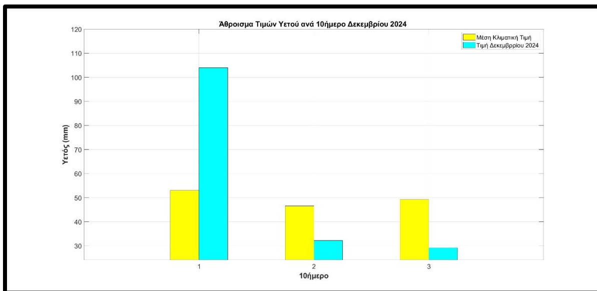
Σχήμα 10. Διακύμανση των αθροιστικών τιμών υετού ανά δεκαήμερο στα Ιωάννινα για το μήνα Δεκέμβριο κατά το έτος 2024. Οι κίτρινες στήλες δείχνουν τις μέσες κλιματικές τιμές, ενώ οι γαλάζιες στήλες τις φετινές τιμές.
