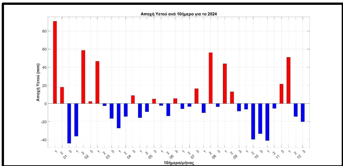
Σχήμα 14. Διακύμανση των αποχών ανά δεκαήμερο (με κόκκινο χρώμα οι θετικές και με μπλε οι αρνητικές) του υετού στα Ιωάννινα (έως και το μήνα Δεκέμβριο) κατά το έτος 2024.
