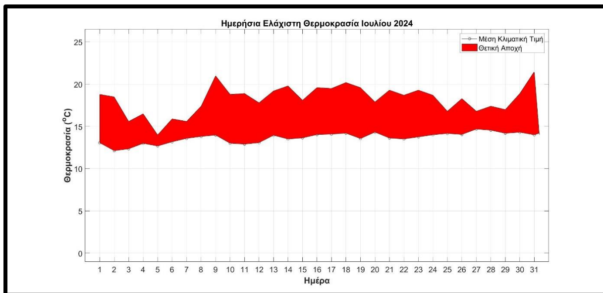
Σχήμα 3. Τιμές ελάχιστης ημερήσιας θερμοκρασίας στα Ιωάννινα για τον Ιούλιο του 2024 και αντίστοιχες μέσες κλιματικές τιμές για τον ίδιο μήνα. Με κόκκινο χρώμα φαίνονται οι θετικές αποχές (διαφορές) των φετινών τιμών από τις κλιματικές.
