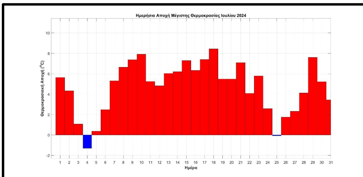
Σχήμα 2. Αποχές (με κόκκινο χρώμα οι θετικές και με μπλε οι αρνητικές) των φετινών από τις μέσες κλιματικές τιμές της μέγιστης ημερήσιας θερμοκρασίας στα Ιωάννινα για το μήνα Ιούλιο, 2024.
