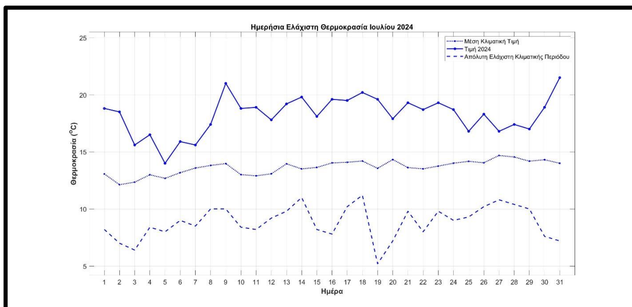
Σχήμα 6. Διακύμανση της ελάχιστης ημερήσιας θερμοκρασίας στα Ιωάννινα κατά το μήνα Ιούλιο του 2024. Η διάστικτη καμπύλη δείχνει τις μέσες κλιματικές τιμές, η διακεκομμένη καμπύλη δείχνει τις απόλυτες ελάχιστες τιμές και η συνεχής καμπύλη με τα σημεία δείχνει τις φετινές τιμές
