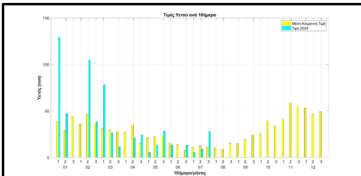
Σχήμα 13. Διακύμανση των αθροιστικών τιμών υετού ανά δεκαήμερο στα Ιωάννινα (έως και το μήνα Ιούλιο) κατά το έτος 2024. Η κίτρινες στήλες δείχνουν τις μέσες κλιματικές τιμές, ενώ οι γαλάζιες στήλες τις φετινές τιμές.
