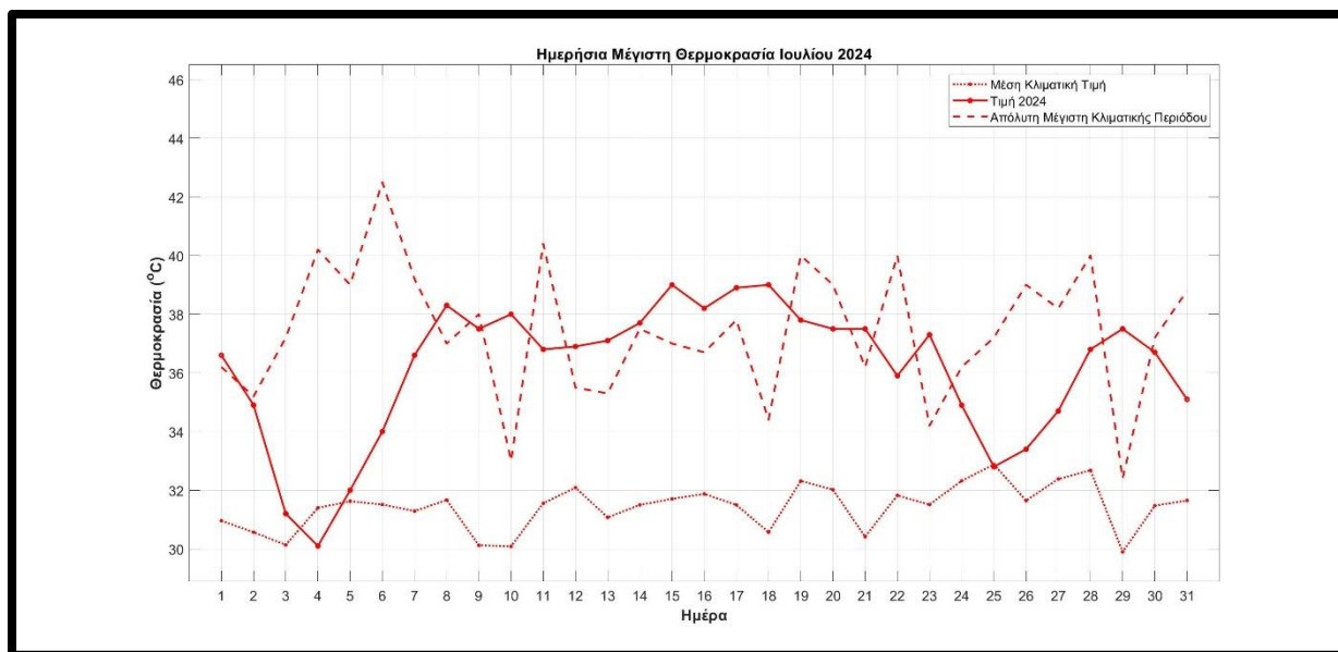
Σχήμα 5. Διακύμανση της μέγιστης ημερήσιας θερμοκρασίας στα Ιωάννινα κατά το μήνα Ιούλιο του 2024. Η διάστικτη καμπύλη δείχνει τις μέσες κλιματικές τιμές, η διακεκομμένη καμπύλη δείχνει τις απόλυτες μέγιστες τιμές και η συνεχής καμπύλη με τα σημεία δείχνει τις φετινές τιμές.
