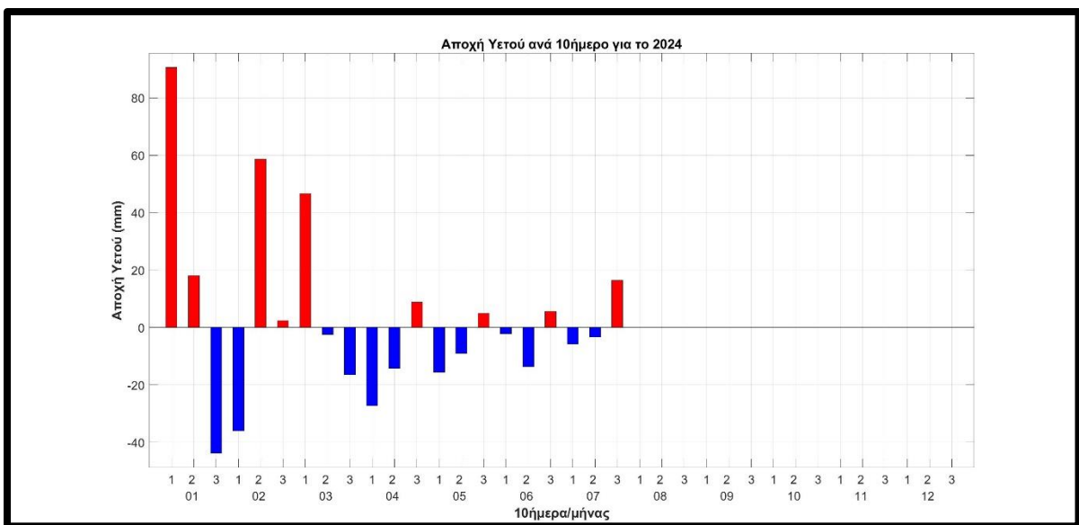
Σχήμα 14. Διακύμανση των αποχών ανά δεκαήμερο (με κόκκινο χρώμα οι θετικές και με μπλε οι αρνητικές) του υετού στα Ιωάννινα (έως και το μήνα Ιούλιο) κατά το έτος 2024.
