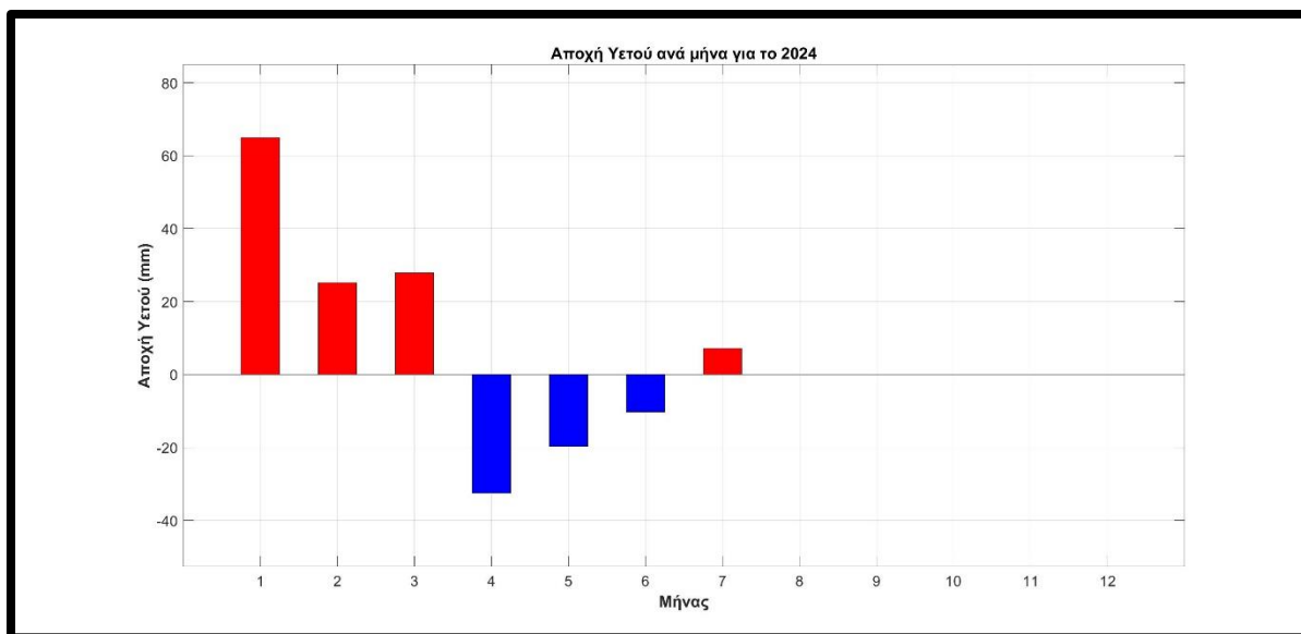
Σχήμα 16. Διακύμανση των αποχών (με κόκκινο χρώμα οι θετικές και με μπλε οι αρνητικές) ανά μήνα του υετού στα Ιωάννινα (έως και το μήνα Ιούλιο) κατά το έτος 2024.
