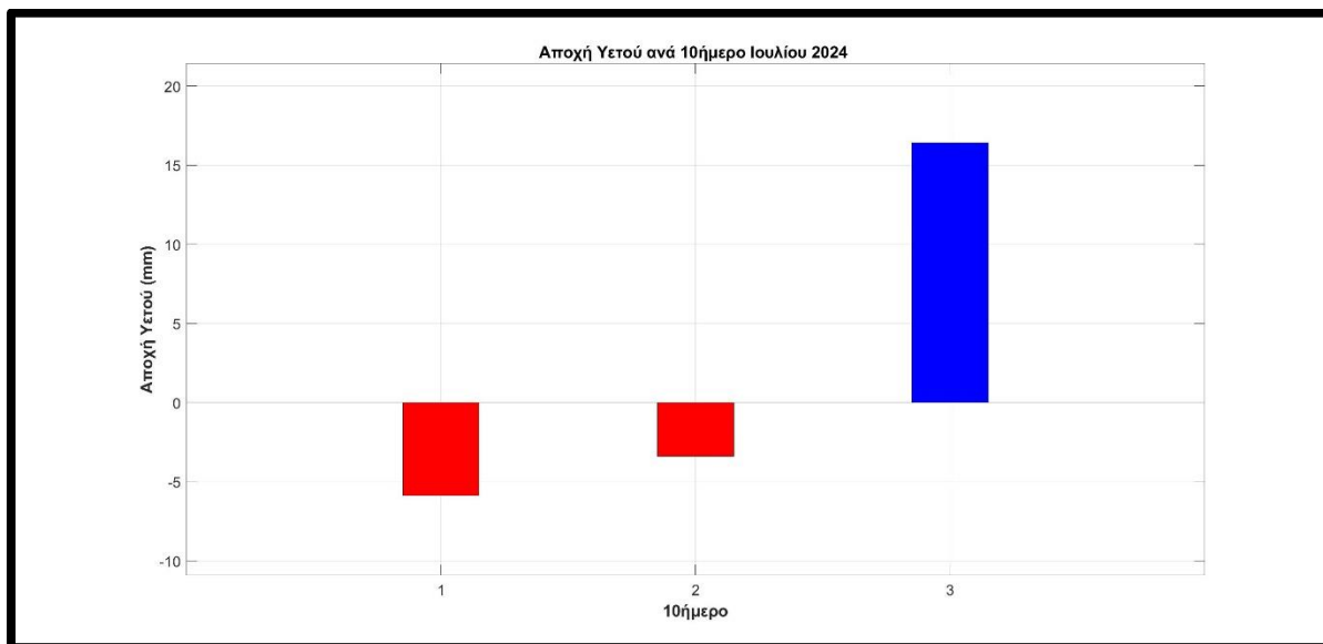
Σχήμα 11. Θετικές αποχές (με κόκκινο χρώμα οι θετικές και με μπλε οι αρνητικές) των φετινών από τις μέσες κλιματικές τιμές των τιμών υετού στα Ιωάννινα για το μήνα Ιούλιο, 2024.
