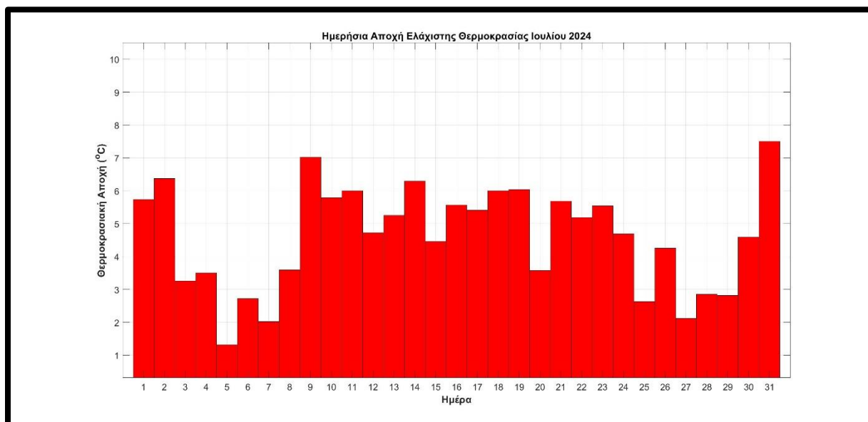
Σχήμα 4. Αποχές (με κόκκινο χρώμα οι θετικές) των φετινών από τις μέσες κλιματικές τιμές της ελάχιστης ημερήσιας θερμοκρασίας στα Ιωάννινα για το μήνα Ιούλιο, 2024.
