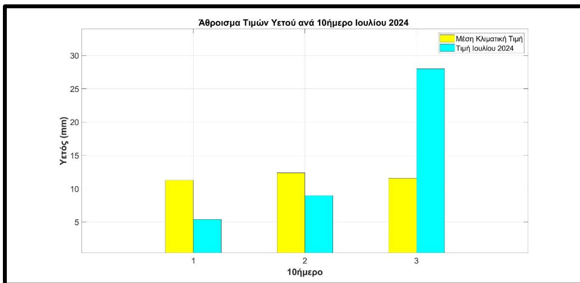
Σχήμα 10. Διακύμανση των αθροιστικών τιμών υετού ανά δεκαήμερο στα Ιωάννινα για το μήνα Ιούλιο κατά το έτος 2024. Οι κίτρινες στήλες δείχνουν τις μέσες κλιματικές τιμές, ενώ οι γαλάζιες στήλες τις φετινές τιμές.
