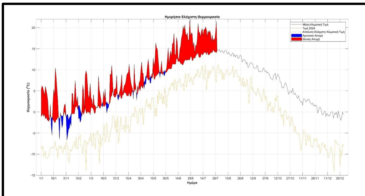
Σχήμα 8. Διακύμανση της ελάχιστης ημερήσιας θερμοκρασίας στα Ιωάννινα (έως και το μήνα Ιούλιο) κατά το έτος 2024. Η μπλε/μαύρη καμπύλη δείχνει τις μέσες κλιματικές τιμές, η πορτοκαλί καμπύλη δείχνει τις απόλυτες ελάχιστες.
