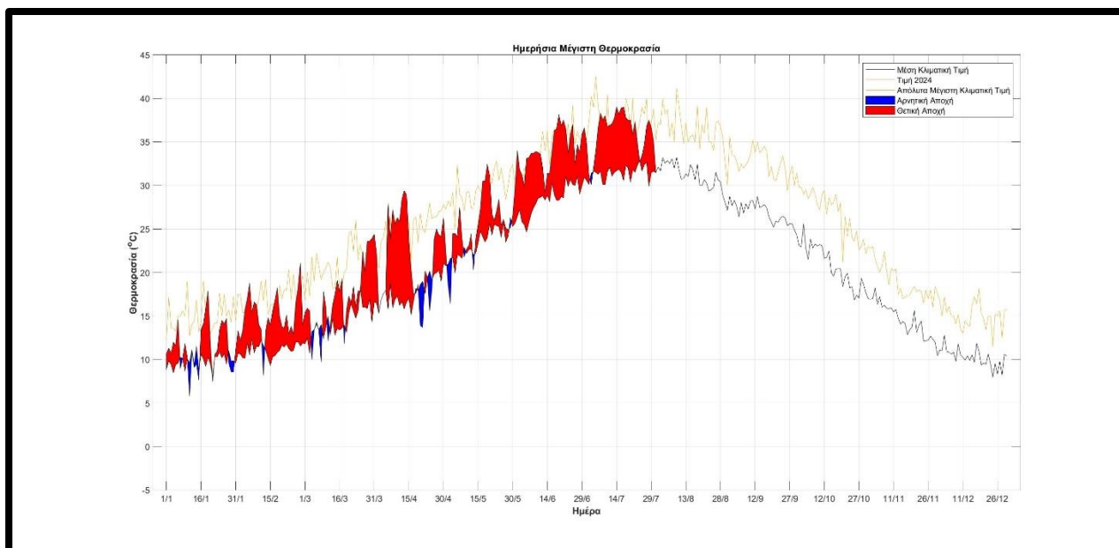
Σχήμα 7. Διακύμανση της μέγιστης ημερήσιας θερμοκρασίας στα Ιωάννινα (έως και το μήνα Ιούλιο) κατά το έτος 2024. Η μπλε/μαύρη καμπύλη δείχνει τις μέσες κλιματικές τιμές, η πορτοκαλί καμπύλη δείχνει τις απόλυτες μέγιστες τιμές.
