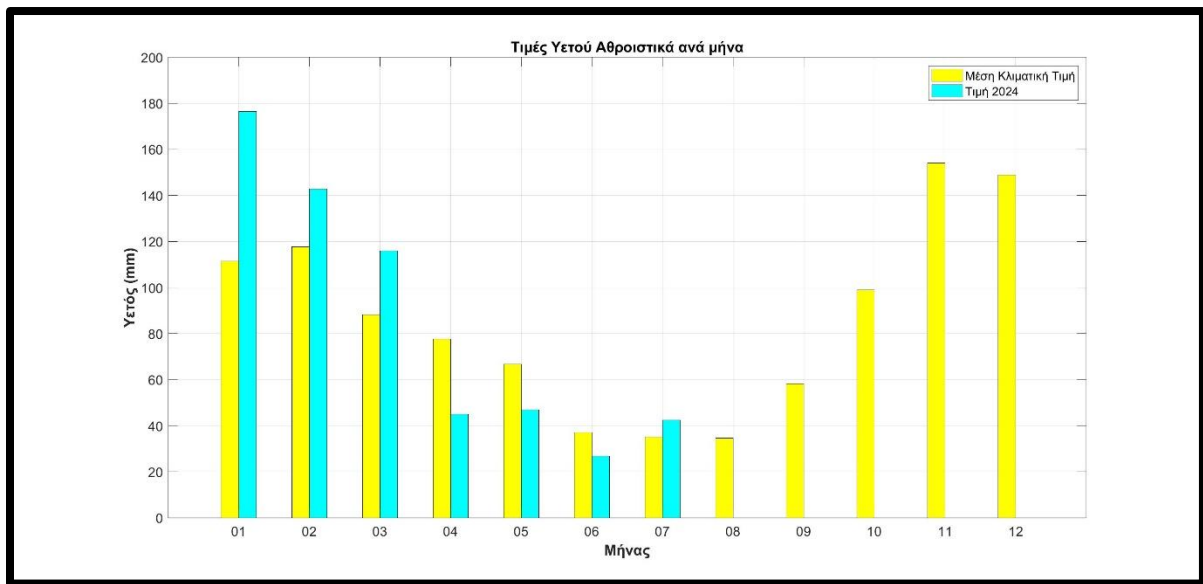
Σχήμα 15. Διακύμανση των τιμών υετού αθροιστικά ανά μήνα στα Ιωάννινα (έως και το μήνα Ιούλιο) κατά το έτος 2024. Η κίτρινη μπάρα δείχνει τις μέσες κλιματικές τιμές, ενώ η γαλάζια μπάρα δείχνει τις φετινές τιμές.
