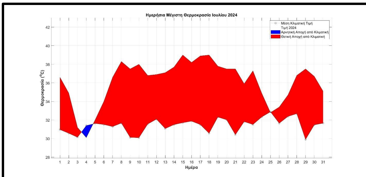
Σχήμα 1. Τιμές μέγιστης ημερήσιας θερμοκρασίας στα Ιωάννινα για τον Ιούλιο του 2024 και αντίστοιχες μέσες κλιματικές τιμές για τον ίδιο μήνα. Με κόκκινο χρώμα φαίνονται οι θετικές αποχές (διαφορές) των φετινών τιμών από τις κλιματικές, ενώ με μπλε χρώμα οι αρνητικές αποχές.
