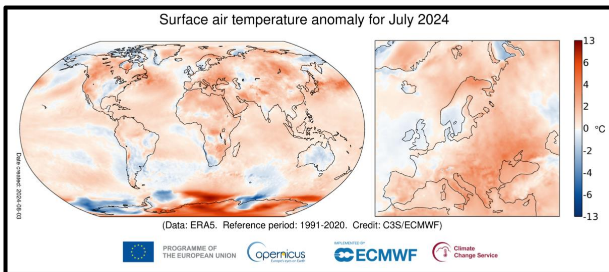
Σχήμα 9. Ανωμαλία (αποχή) της επιφανειακής θερμοκρασίας για τη Γη (αριστερά) και την Ευρώπη (δεξιά) κατά τον Ιούλιο του 2024 (Πηγή: Copernicus Atmospheric Monitoring Service, CAMS).
