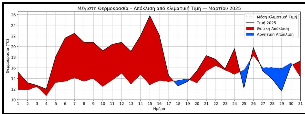
Σχήμα 1. Τιμές μέγιστης ημερήσιας θερμοκρασίας στα Ιωάννινα για τον Μάρτιο του 2025 και αντίστοιχες μέσες κλιματικές τιμές για τον ίδιο μήνα. Με κόκκινο χρώμα φαίνονται οι θετικές αποχές (διαφορές) των φετινών τιμών από τις κλιματικές, ενώ με μπλε χρώμα οι αρνητικές αποχές.
