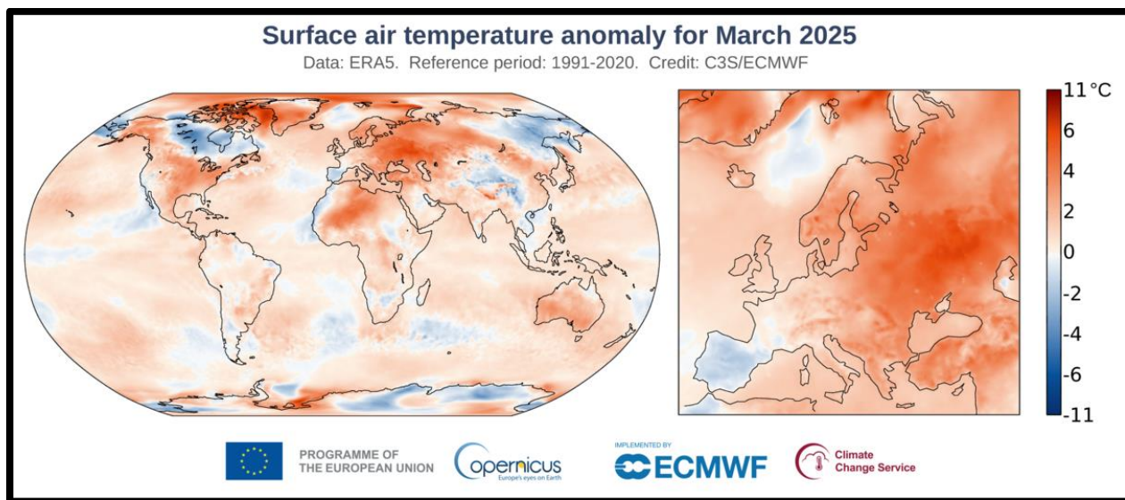
Σχήμα 9. Ανωμαλία (αποχή) της επιφανειακής θερμοκρασίας για τη Γη (αριστερά) και την Ευρώπη (δεξιά) κατά τον Μάρτιο του 2025 (Πηγή: Copernicus Atmospheric Monitoring Service, CAMS).
