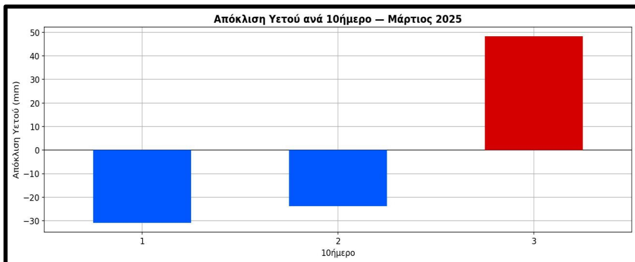
Σχήμα 11. Αποχές (με κόκκινο χρώμα οι θετικές και με μπλε οι αρνητικές) ανά δεκαήμερο των φετινών από τις μέσες κλιματικές τιμές των τιμών υετού στα Ιωάννινα για το μήνα Μάρτιο του 2025.
