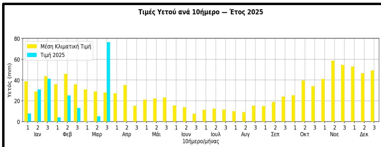
Σχήμα 13. Διακύμανση των αθροιστικών τιμών υετού ανά δεκαήμερο στα Ιωάννινα, έως και το μήνα Μάρτιο, κατά το έτος 2025. Οι κίτρινες στήλες δείχνουν τις μέσες κλιματικές τιμές, ενώ οι γαλάζιες στήλες τις τιμές του 2025.
