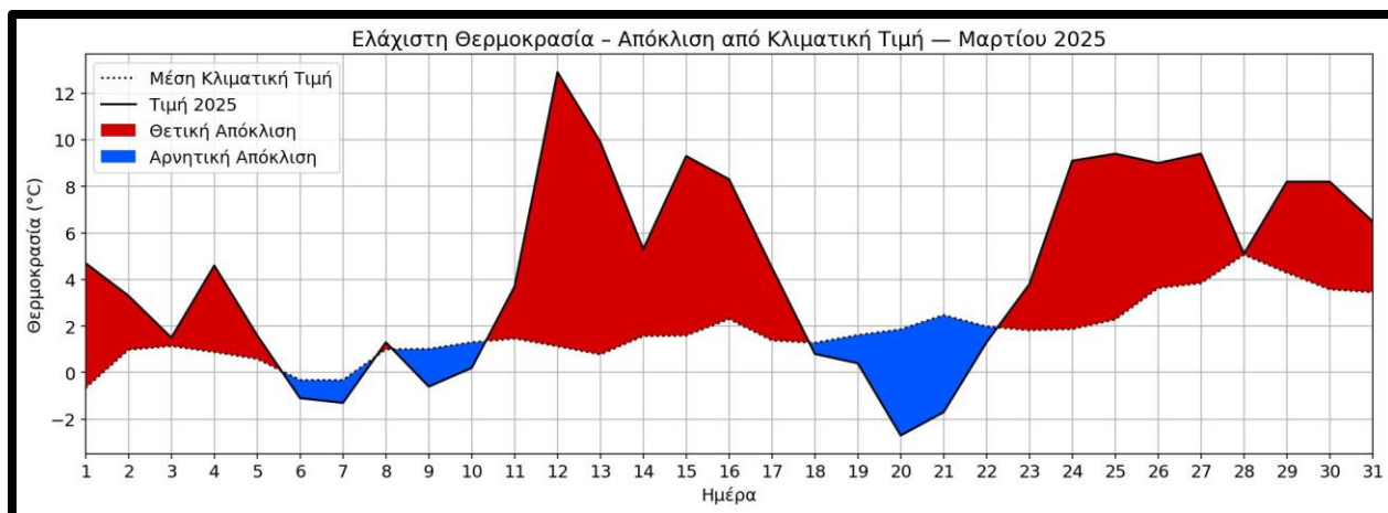
Σχήμα 3. Τιμές ελάχιστης ημερήσιας θερμοκρασίας στα Ιωάννινα για τον Μάρτιο του 2025 και αντίστοιχες μέσες κλιματικές τιμές για τον ίδιο μήνα. Με κόκκινο χρώμα φαίνονται οι θετικές αποχές (διαφορές) των φετινών τιμών από τις κλιματικές, ενώ με μπλε χρώμα οι αρνητικές αποχές.
