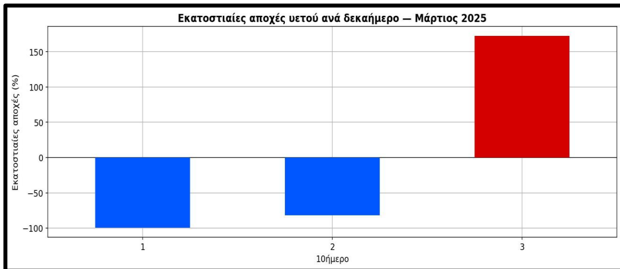
Σχήμα 12. Εκατοστιαίες απόλυτες αποχές (με κόκκινο χρώμα οι θετικές και με μπλε οι αρνητικές) ανά δεκαήμερο για το μήνα Μάρτιο του 2025.
