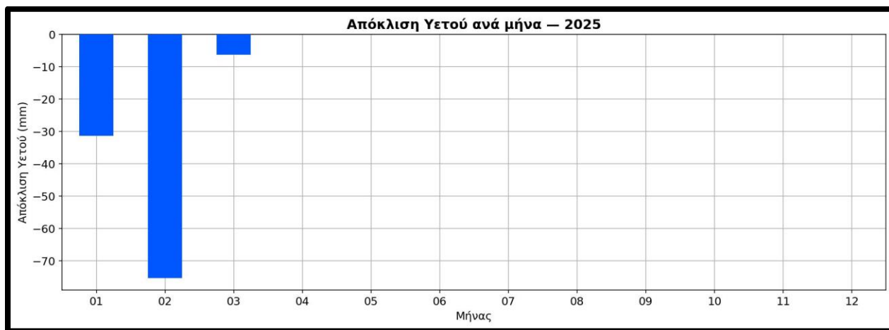
Σχήμα 16. Διακύμανση των αποχών ανά μήνα (με κόκκινο χρώμα οι θετικές και με μπλε οι αρνητικές) του υετού στα Ιωάννινα, έως και το μήνα Μάρτιο, κατά το έτος 2025.
