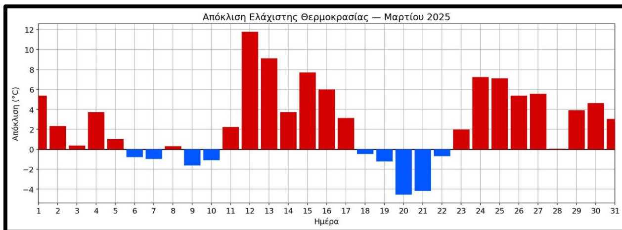
Σχήμα 4. Αποχές (με κόκκινο χρώμα οι θετικές και με μπλε οι αρνητικές) των φετινών από τις μέσες κλιματικές τιμές της ελάχιστης ημερήσιας θερμοκρασίας στα Ιωάννινα για το μήνα Μάρτιο του 2025.
