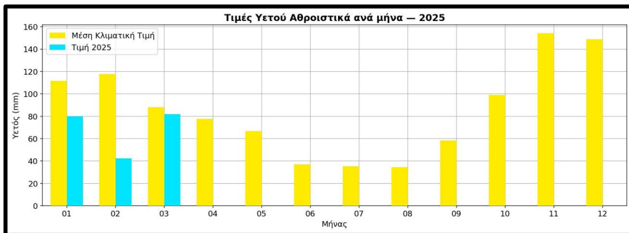
Σχήμα 15. Διακύμανση των αθροιστικών τιμών υετού ανά μήνα στα Ιωάννινα, έως και το μήνα Μάρτιο, κατά το έτος 2025. Οι κίτρινες στήλες αντιστοιχούν στις μέσες κλιματικές τιμές, ενώ οι γαλάζιες στις τιμές του 2025.
