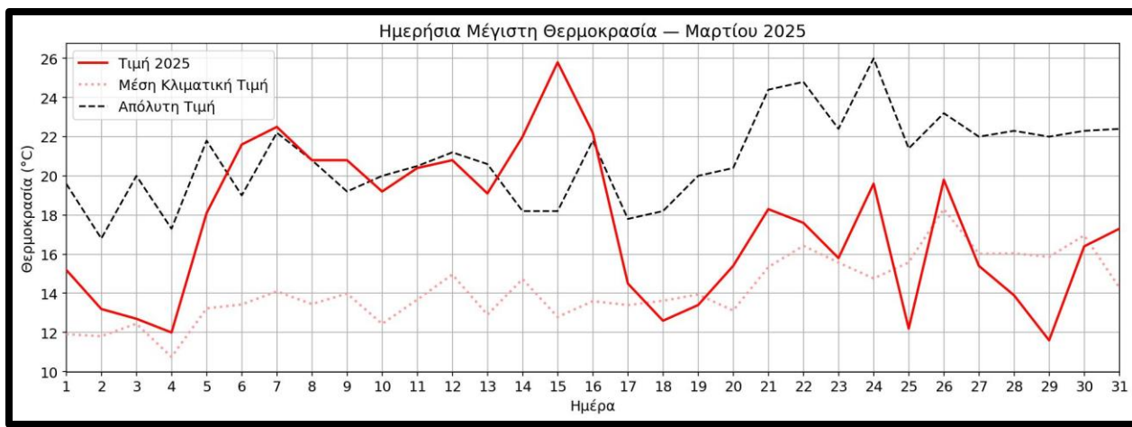
Σχήμα 5. Διακύμανση της μέγιστης ημερήσιας θερμοκρασίας στα Ιωάννινα κατά το μήνα Μάρτιο του 2025. Η διάστικτη καμπύλη δείχνει τις μέσες κλιματικές τιμές, η διακεκομμένη καμπύλη δείχνει τις απόλυτες μέγιστες τιμές (θερμοκρασίες ρεκόρ ανά ημέρα) και η συνεχής καμπύλη με τα σημεία δείχνει τις φετινές τιμές.
