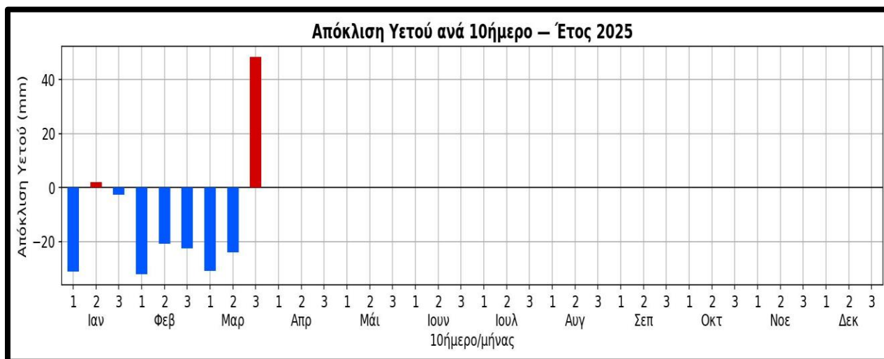
Σχήμα 14. Διακύμανση των αποχών ανά δεκαήμερο (με κόκκινο χρώμα οι θετικές και με μπλε οι αρνητικές) του υετού στα Ιωάννινα, έως και το μήνα Μάρτιο, κατά το έτος 2025.
