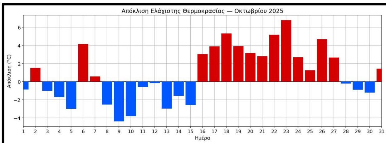
Σχήμα 4. Αποχές (με κόκκινο χρώμα οι θετικές και με μπλε οι αρνητικές) των φετινών από τις μέσες κλιματικές τιμές της ελάχιστης ημερήσιας θερμοκρασίας στα Ιωάννινα για το μήνα Οκτώβριο του 2025.
