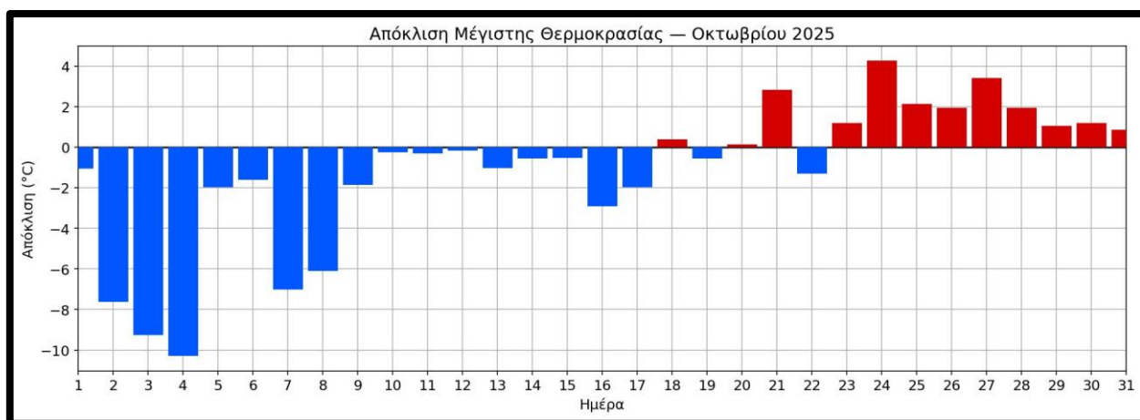
Σχήμα 2. Αποχές (με κόκκινο χρώμα οι θετικές και με μπλε οι αρνητικές) των φετινών από τις μέσες κλιματικές τιμές της μέγιστης ημερήσιας θερμοκρασίας στα Ιωάννινα για το μήνα Οκτώβριο του 2025.
