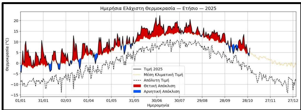
Σχήμα 8. Διακύμανση της ελάχιστης ημερήσιας θερμοκρασίας στα Ιωάννινα (έως και το μήνα Οκτώβριο) κατά το έτος 2025. Η μπλε/μαύρη καμπύλη δείχνει τις μέσες κλιματικές τιμές, η πορτοκαλί καμπύλη δείχνει τις απόλυτες ελάχιστες.
