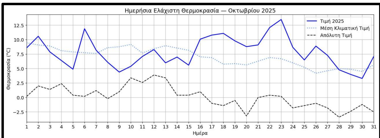
Σχήμα 6. Διακύμανση της ελάχιστης ημερήσιας θερμοκρασίας στα Ιωάννινα κατά το μήνα Οκτώβριο του 2025. Η διάστικτη καμπύλη δείχνει τις μέσες κλιματικές τιμές, η διακεκομμένη καμπύλη δείχνει τις απόλυτες ελάχιστες τιμές και η συνεχής καμπύλη με τα σημεία δείχνει τις φετινές τιμές.
