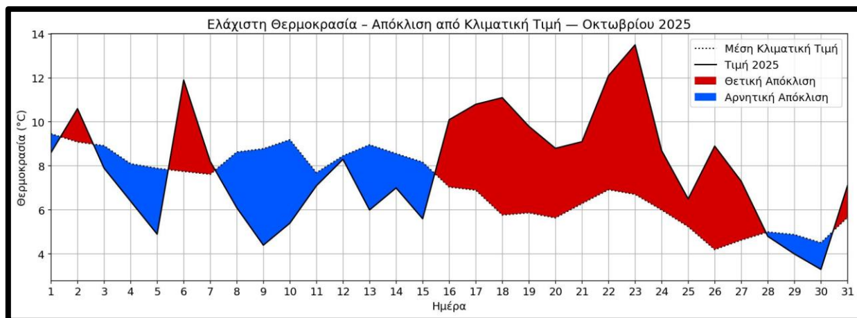
Σχήμα 3. Τιμές ελάχιστης ημερήσιας θερμοκρασίας στα Ιωάννινα για τον Οκτώβριο του 2025 και αντίστοιχες μέσες κλιματικές τιμές για τον ίδιο μήνα. Με κόκκινο χρώμα φαίνονται οι θετικές αποχές (διαφορές) των φετινών τιμών από τις κλιματικές, ενώ με μπλε χρώμα οι αρνητικές αποχές.
