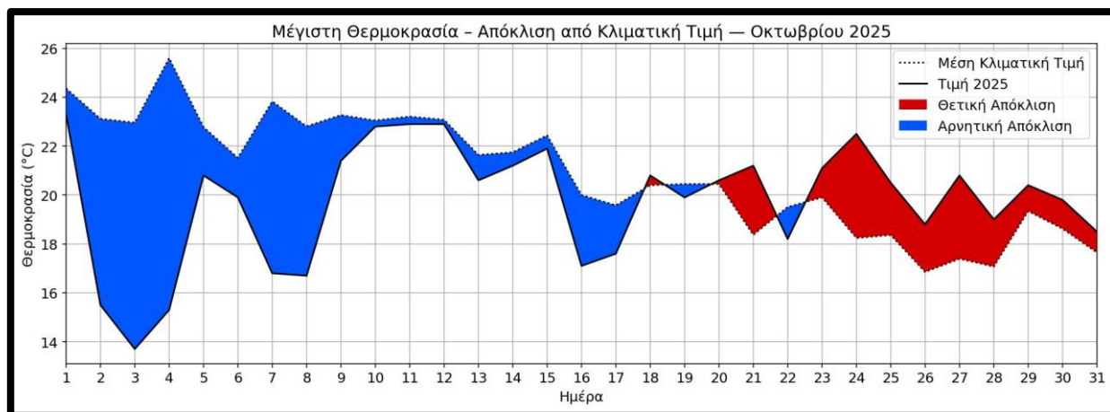
Σχήμα 1. Τιμές μέγιστης ημερήσιας θερμοκρασίας στα Ιωάννινα για τον Οκτώβριο του 2025 και αντίστοιχες μέσες κλιματικές τιμές για τον ίδιο μήνα. Με κόκκινο χρώμα φαίνονται οι θετικές αποχές (διαφορές) των φετινών τιμών από τις κλιματικές, ενώ με μπλε χρώμα οι αρνητικές αποχές.
