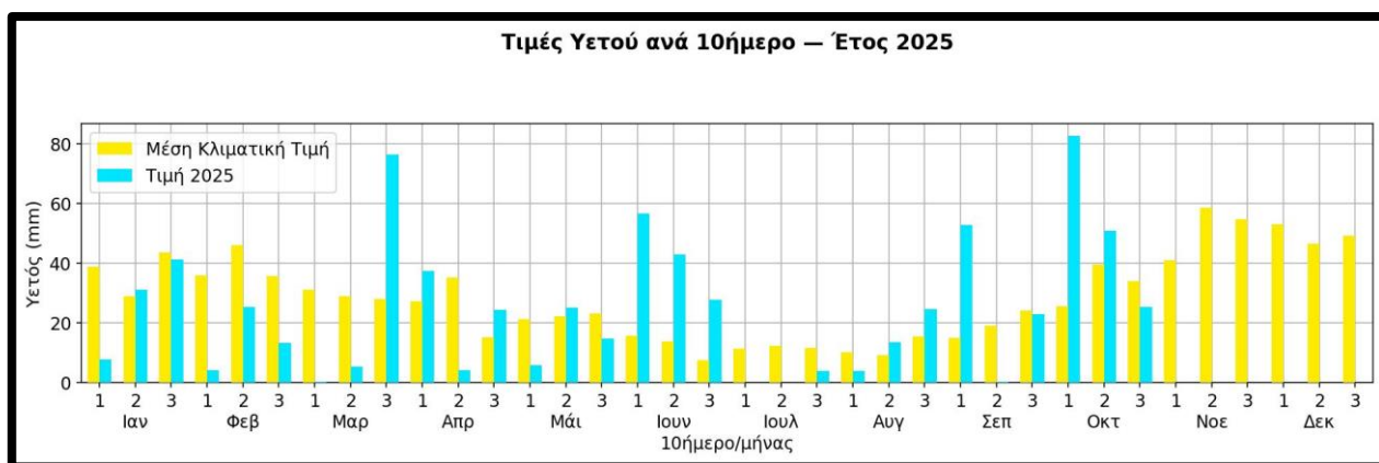
Σχήμα 13. Διακύμανση των αθροιστικών τιμών υετού ανά δεκαήμερο στα Ιωάννινα (έως και το μήνα Οκτώβριο) κατά το έτος 2025. Οι κίτρινες στήλες δείχνουν τις μέσες κλιματικές τιμές, ενώ οι γαλάζιες στήλες τις φετινές τιμές.
