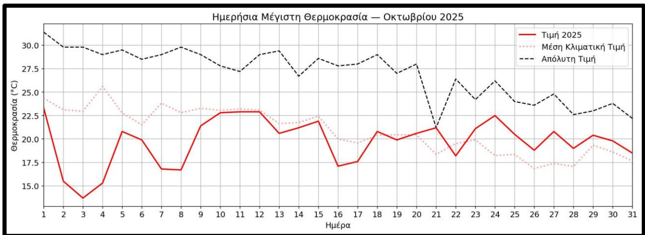
Σχήμα 5. Διακύμανση της μέγιστης ημερήσιας θερμοκρασίας στα Ιωάννινα κατά το μήνα Οκτώβριο του 2025. Η διάστικτη καμπύλη δείχνει τις μέσες κλιματικές τιμές, η διακεκομμένη καμπύλη δείχνει τις απόλυτες μέγιστες τιμές και η συνεχής καμπύλη με τα σημεία δείχνει τις φετινές τιμές.
